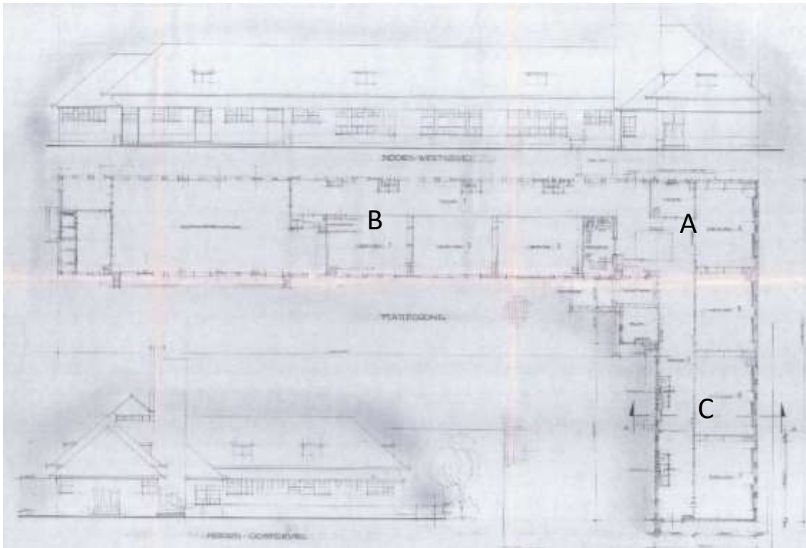
6 – Plattegrond bestaande situatie in 1983 met hoofdvolume (A), westvleugel (B) en zuidvleugel (C)
